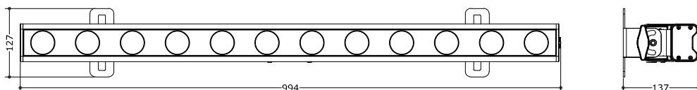
Disegno tecnico
